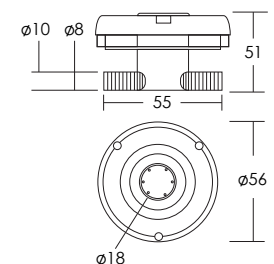
Face & Barb Jet
